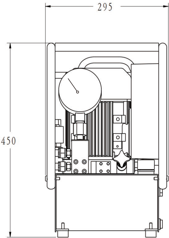
▼ EPA 外形尺寸图:
