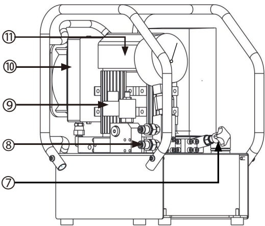
▼ EPA1500 产品示意图:
