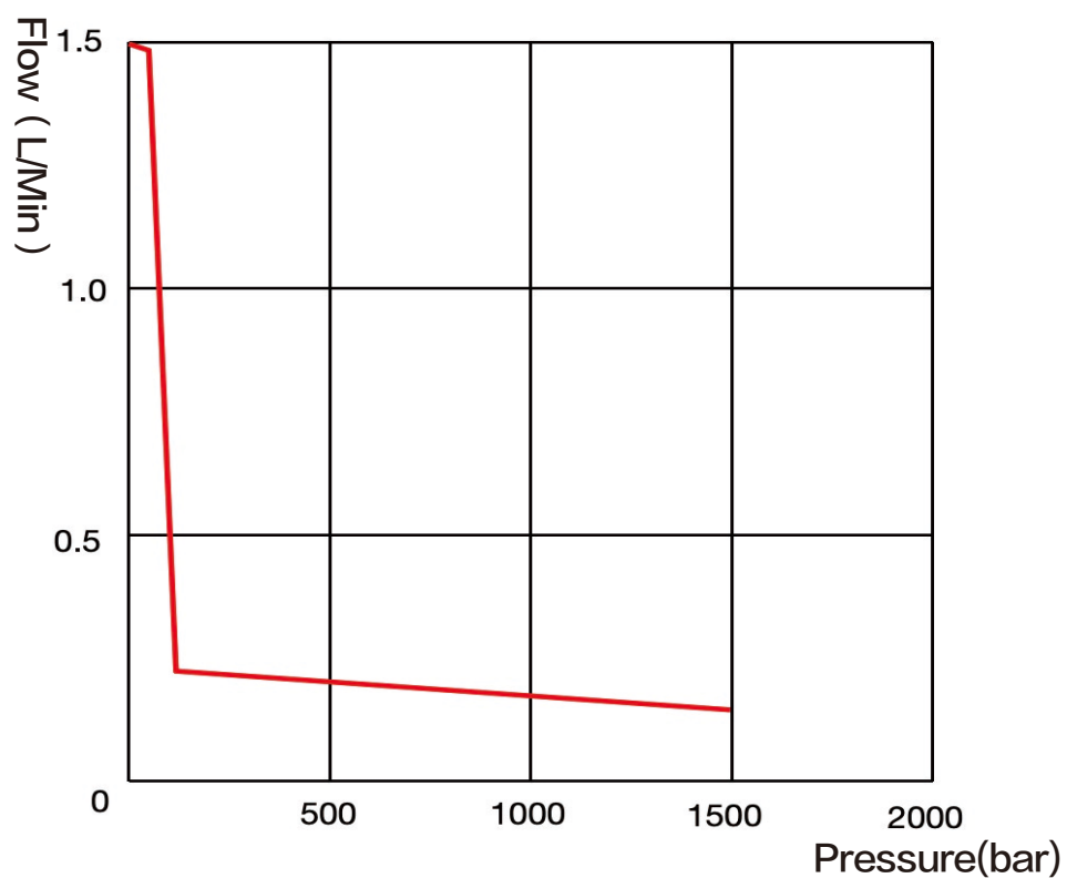
▼ EPA1500 压力流量图：
