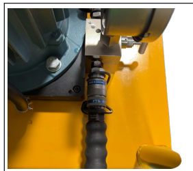
推入油管后，将外锁环前推，顺时针旋转锁定。
