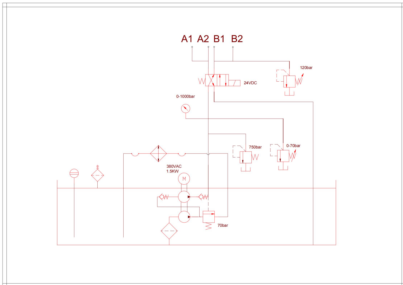
▼ EX-HE5TW 液压原理图:
