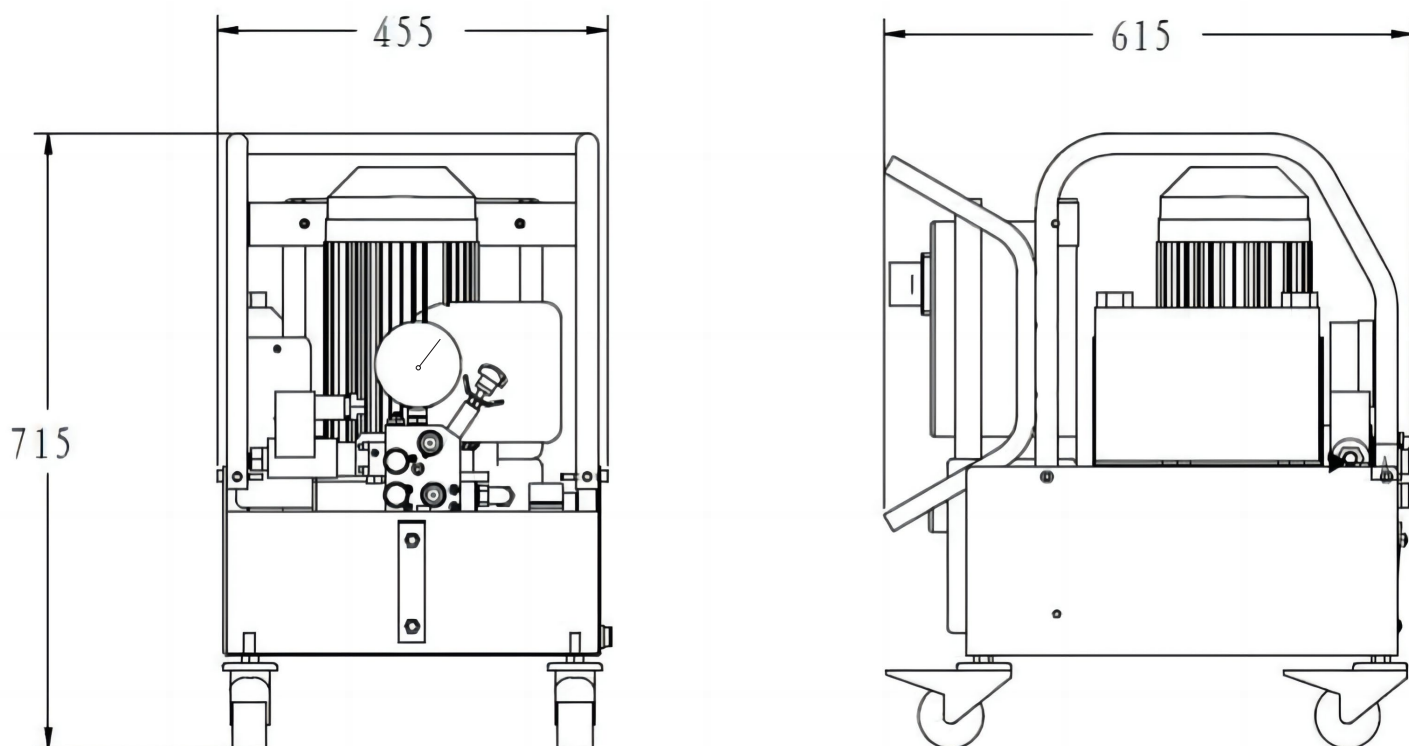
▼ EX-HE5TW 外形尺寸图:
