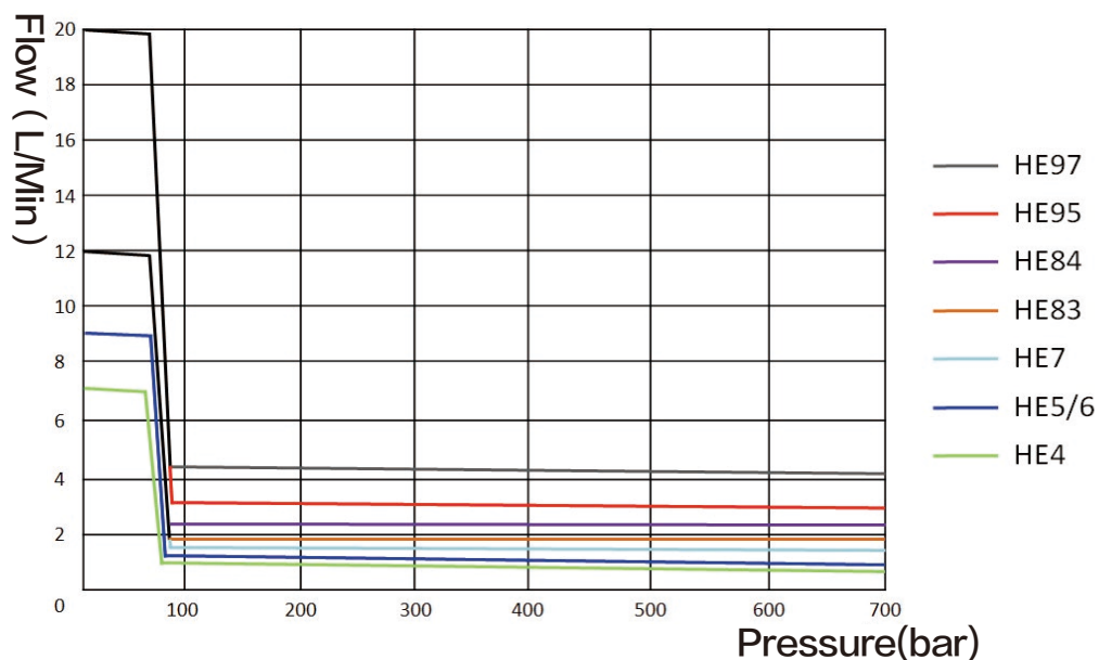
HE 系列电动泵压力与流量曲线图
