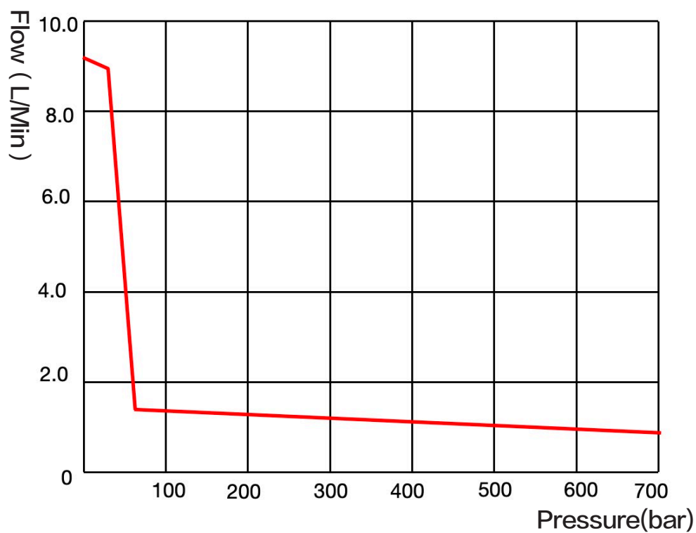
▼ HE5TW10-AT 压力流量图:
