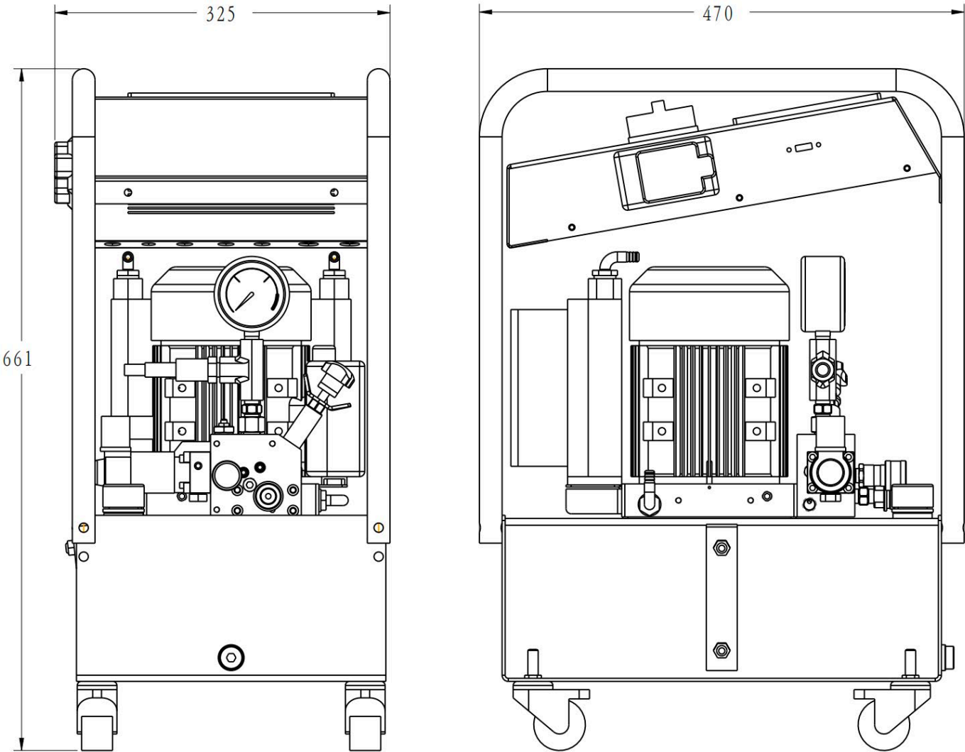
▼ HE5TW10-AT 产品外形图：
