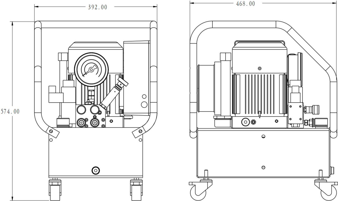
▼ HE7TW10 外形尺寸图：
