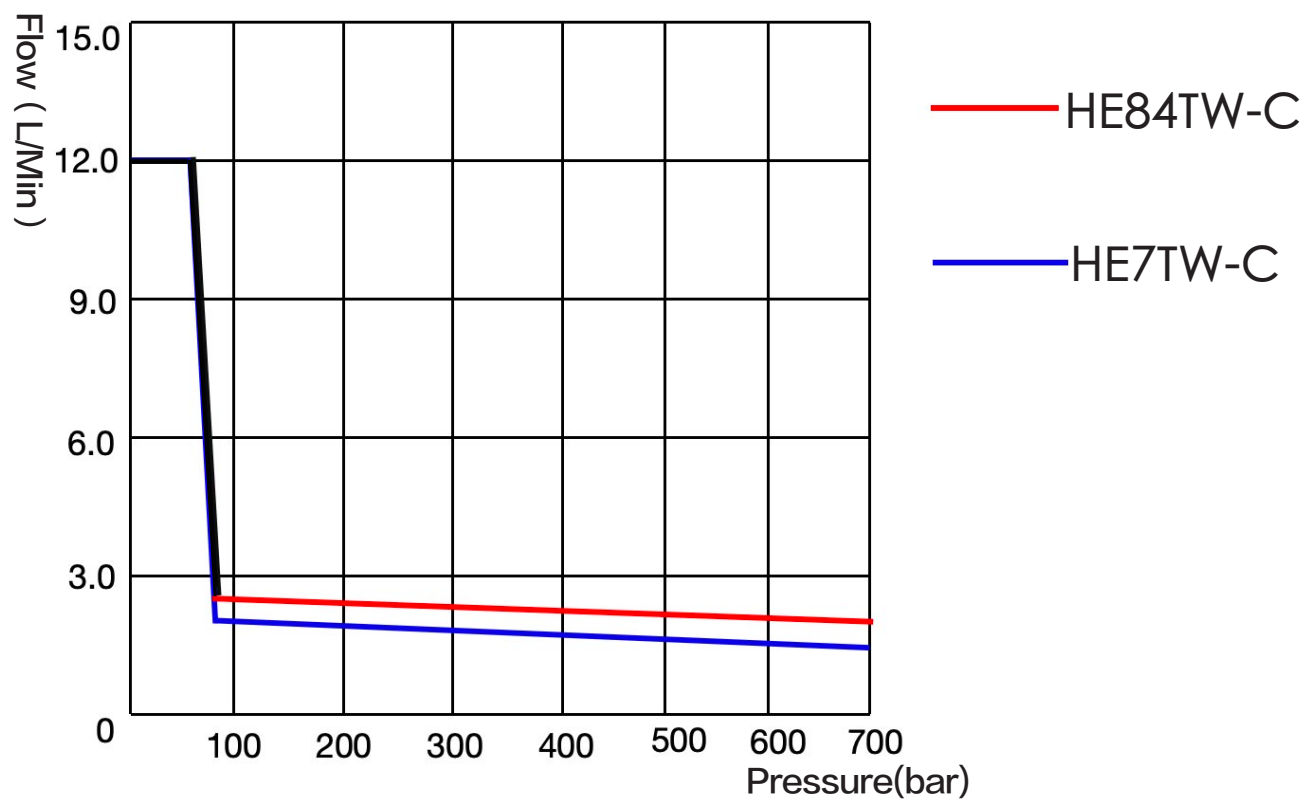
▼ HETW-C 压力流量图：
