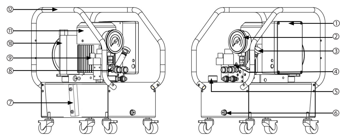
▼ HE7TW10 产品示意图：
